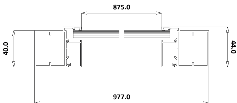
SEZIONE AA
