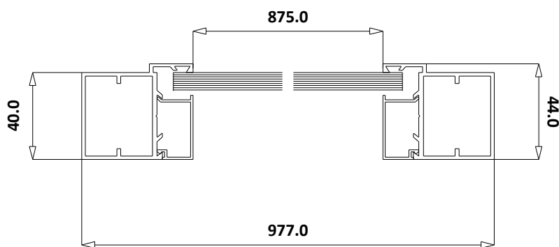
SEZIONE AA
