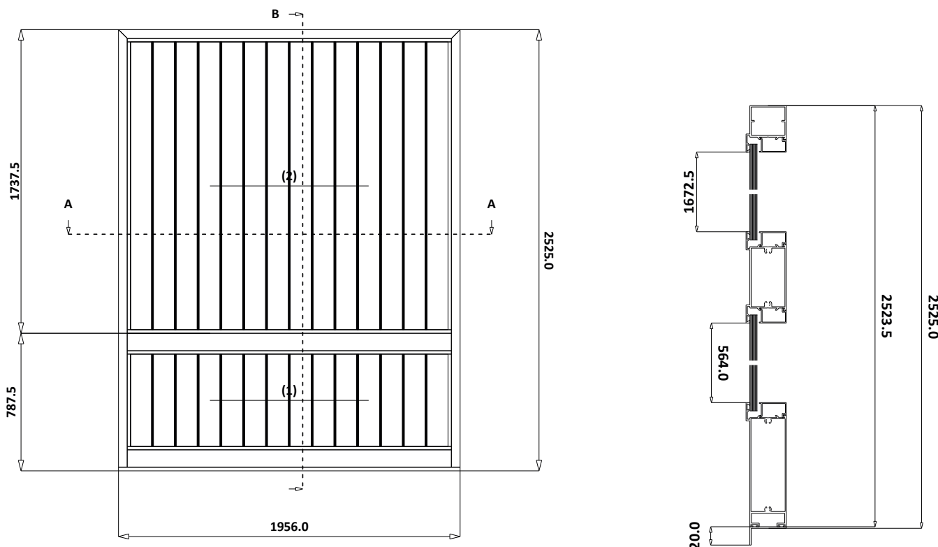
SEZIONE BB
